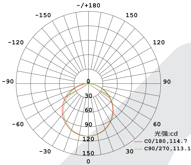
配光曲线
